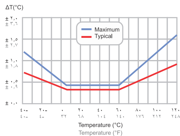
نمودار تغییرات خطای دما و رطوبت
